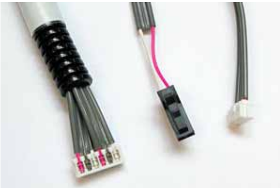
A500662 - Cable EKM ACO312 + FF SE11 (2.4m)
